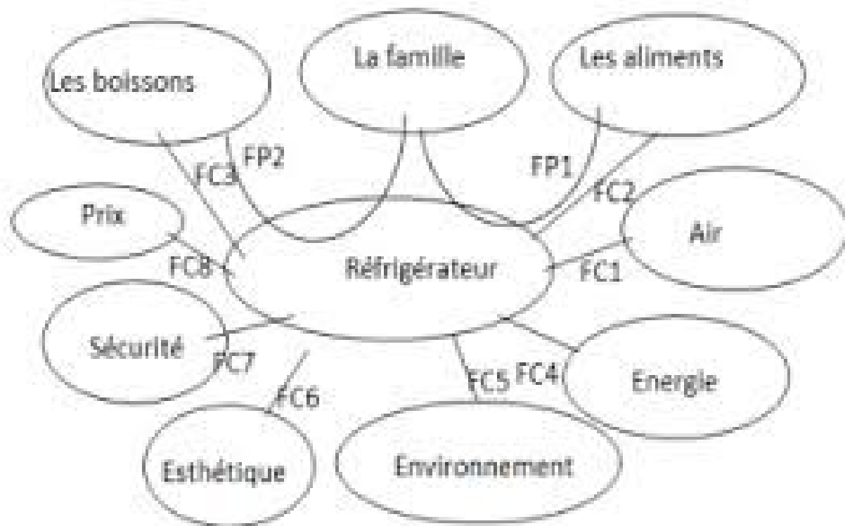
Diagramme pieuvre (graphe des interacteurs)
